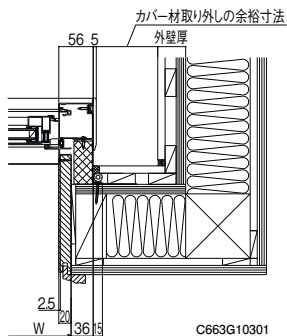
〈入隅の納まり〉 W 36.5 C663G10301
